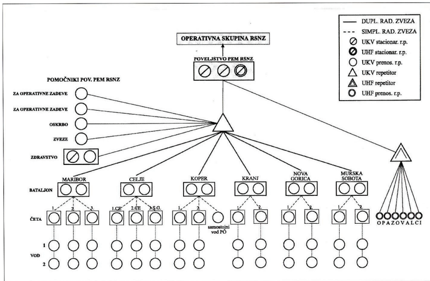
Slika 3: Sistem zvez v akciji »Sever« (Bukovnik, 2002: 137)
